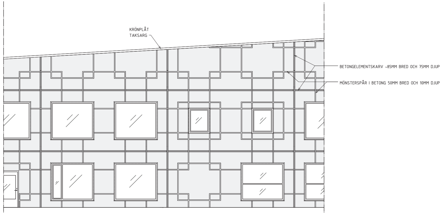
FASADUTSNITT BETONGELEMENT SKALA 1:50
