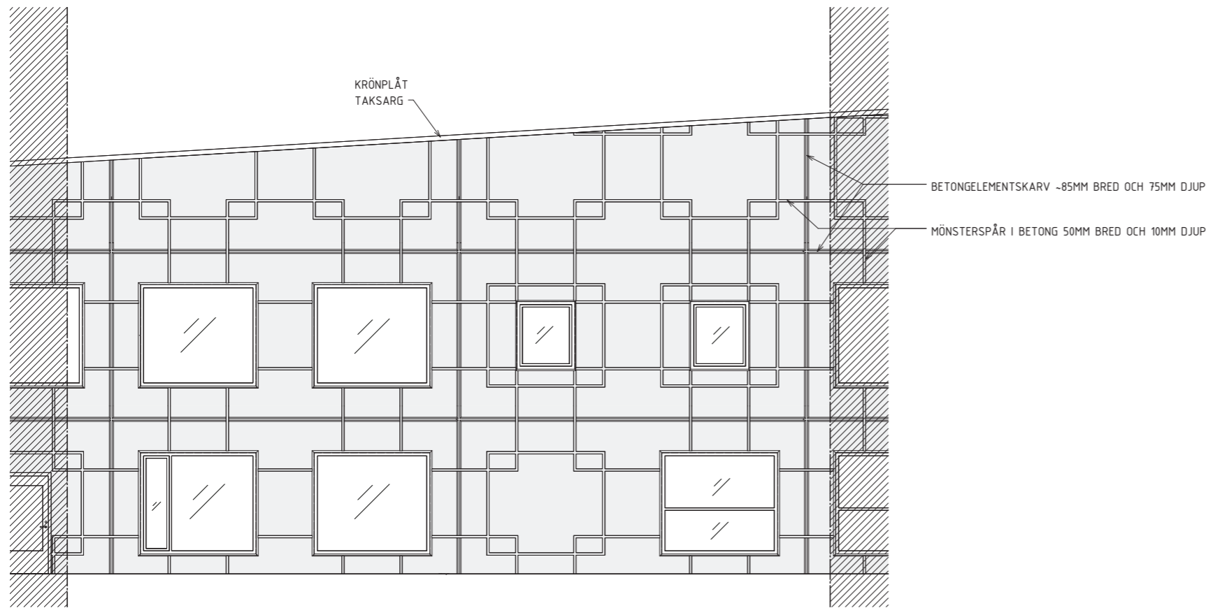
FASADUTSNITT BETONGELEMENT SKALA 1:50
